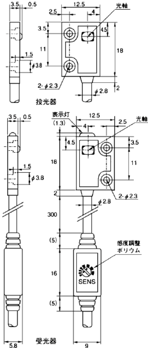
センサー外形図
