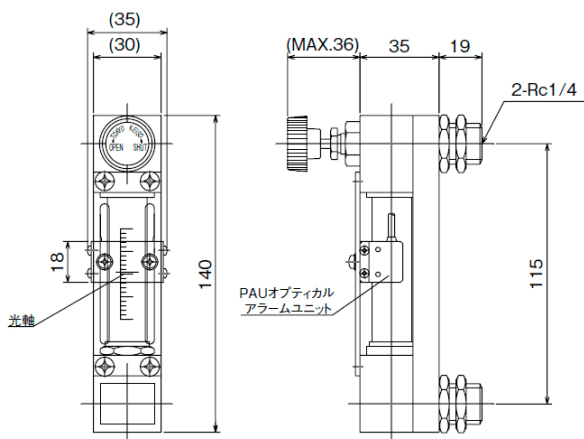
組付外形図 (P-100-UE-4N-R2)
