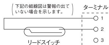
結線図
