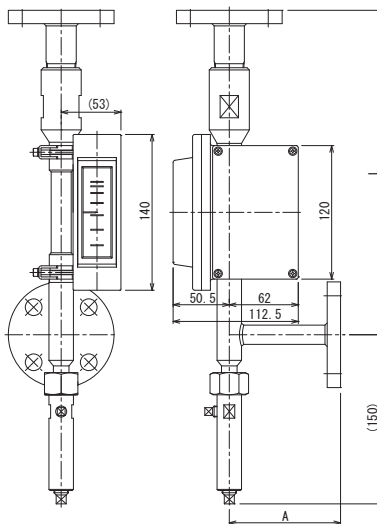
大流量タイプ、フランジ接続
