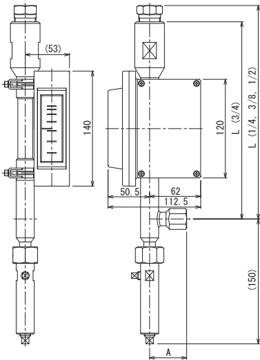
大流量タイプ、ねじ接続
