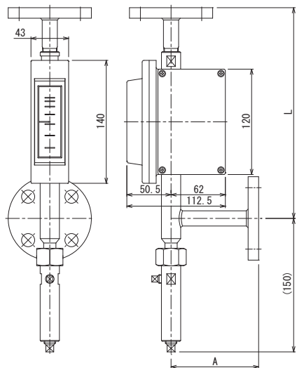
標準タイプ、フランジ接続
