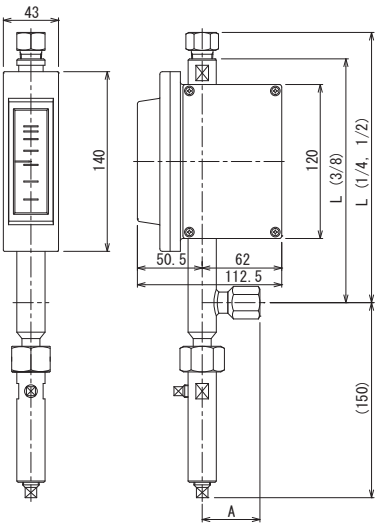
標準タイプ、ねじ接続
