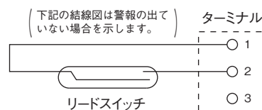
結線図
