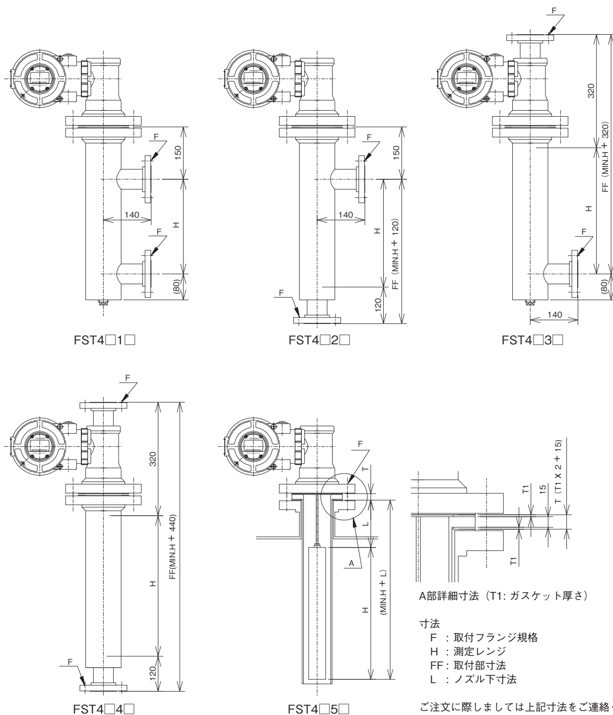
●図2 チャンパ取り付け方法（# 150, # 300 寸法、図は左側取付を示す）
