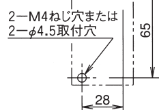
取付穴寸法図 (ねじ取付けの場合)
