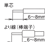
電線の端末処理
