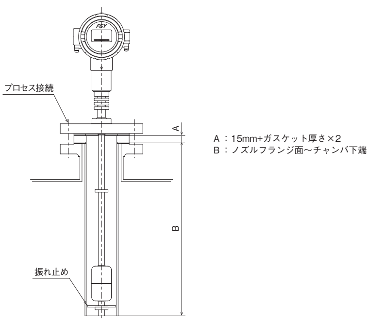
図4 外形図(内筒チャンバの場合)
