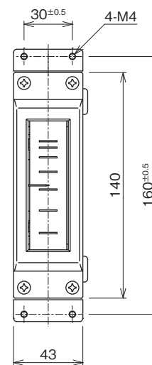
●パネル取付構造 (正面側)
