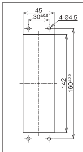
●パネルカット寸法図
