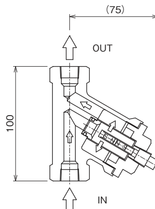
●マグネットストレーナ 外形寸法図
