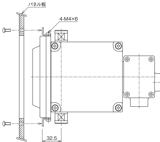
●パネル取付構造 (側面側)
