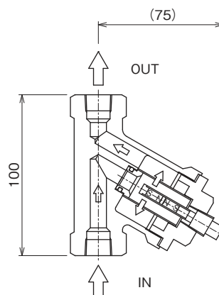
●マグネットストレーナ 外形寸法図
