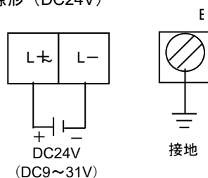
DC24V (DC9~31V)
