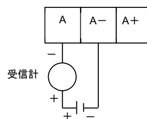
外部電源 (DC32V以下)
