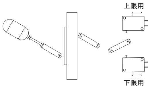
反発式・放熱フィン付
