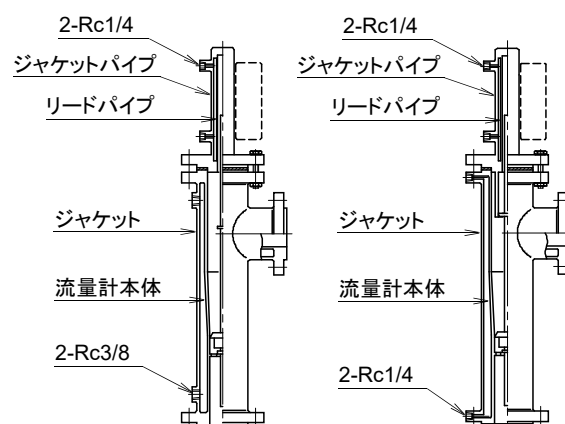
断熱ジャケット装着品 AM7□□□/J□
