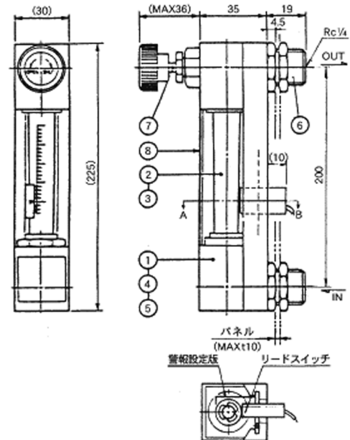
【P-200-U A/B/C/D 標準外形図】
