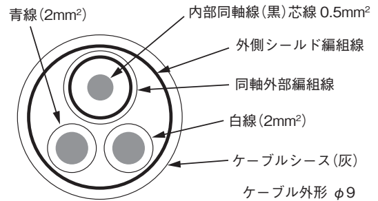
図6.1 ケーブル構造
