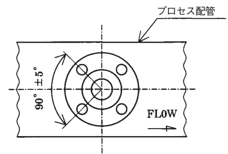
●検出器取付フランジ図
