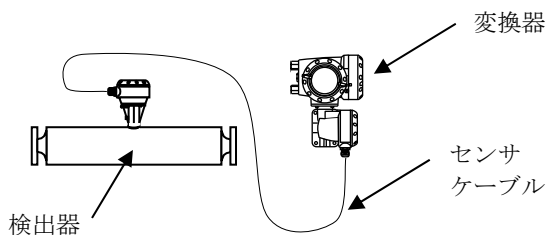
MMS1000F,2000F,7000F 検出器 MMC400F 変換器 (分離形・オプション 代表例)
