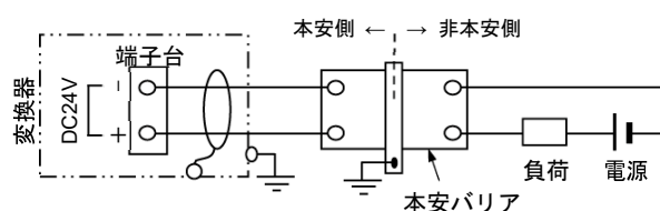
図-18 本質安全防爆構造の結線ループ図 (MTL7728+を使用の場合)
