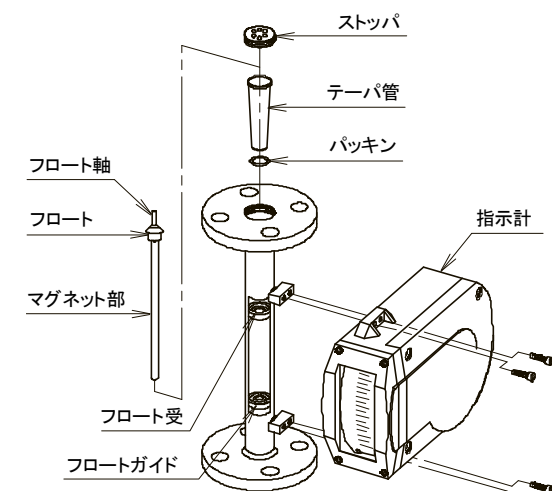
メータサイズ 15 (標準タイプ)
