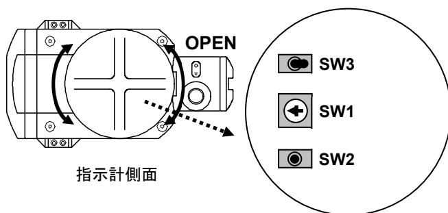
SW1：ロータリースイッチ SW2：押しボタンスイッチ SW3：トグルスイッチ
