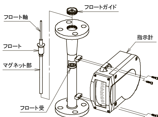
メータサイズ 20~50
