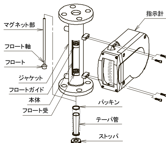
メータサイズ 15(高粘度タイプ)
